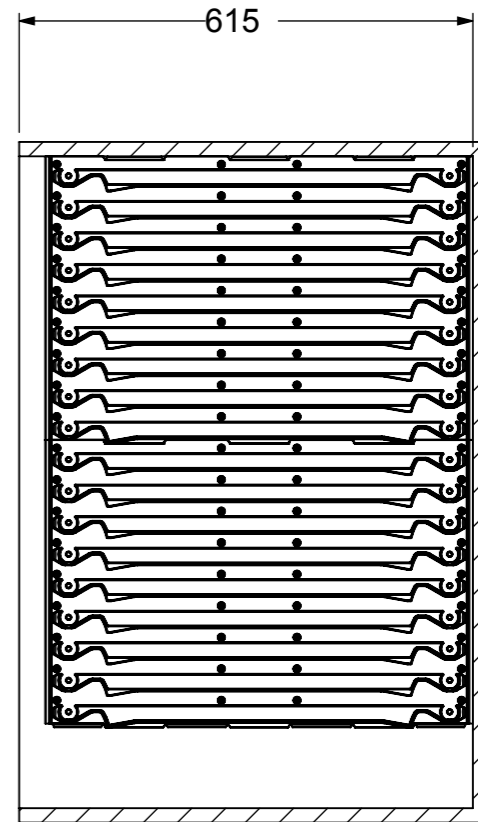
SECTION D-D
